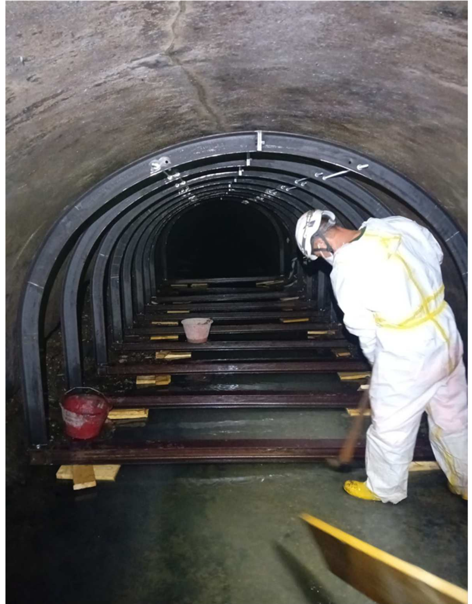
MESSA IN SICUREZZA PER L'ESECUZIONE DEI LAVORI MEDIANTE POSA DI CENTINE METALLICHE REALIZZATE SU MISURA
